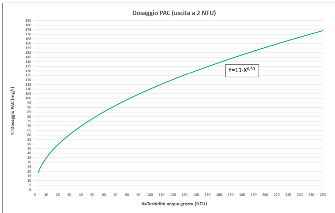
Figura 1 – Curva requisiti prestazionali minimi
