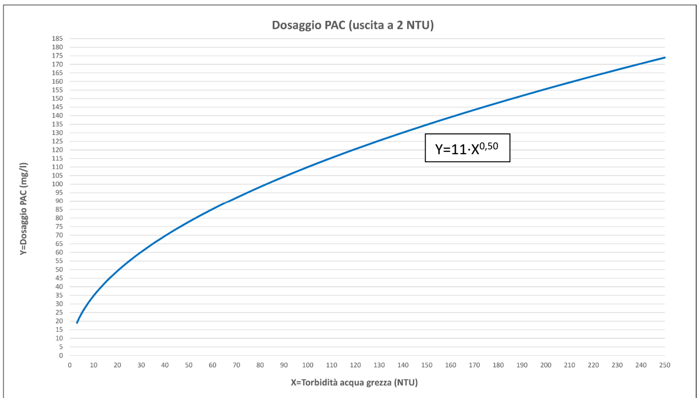
Figura 1 – Curva requisiti prestazionali minimi
